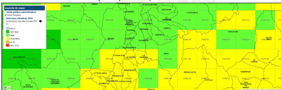
Ilustración 6. Amenaza para temperaturas muy altas. Escenarios RCP 4.5 2016 - 2040
