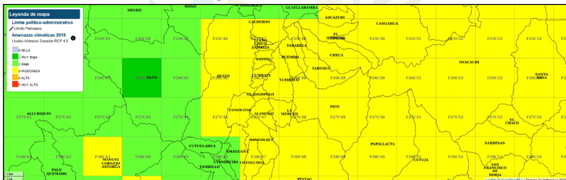
Ilustración 3. Amenaza para lluvias intensas. Escenarios RCP 4.5 2016 - 2040
