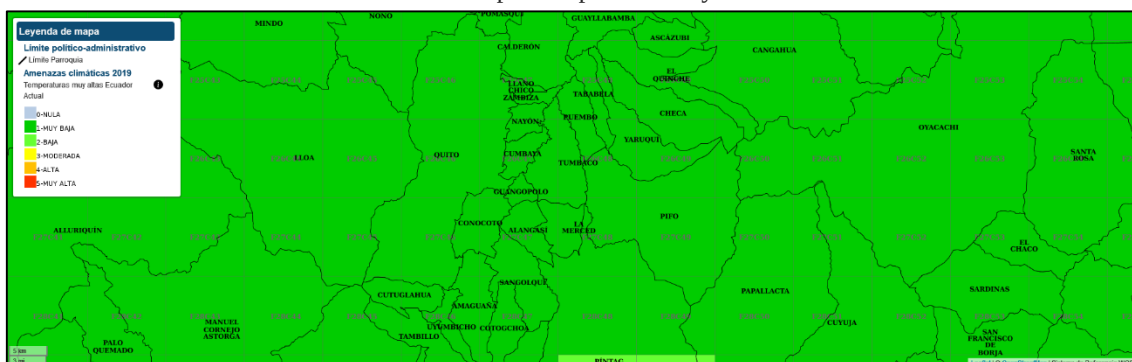
Ilustración 5. Amenaza para temperaturas muy altas 1981 - 2015
