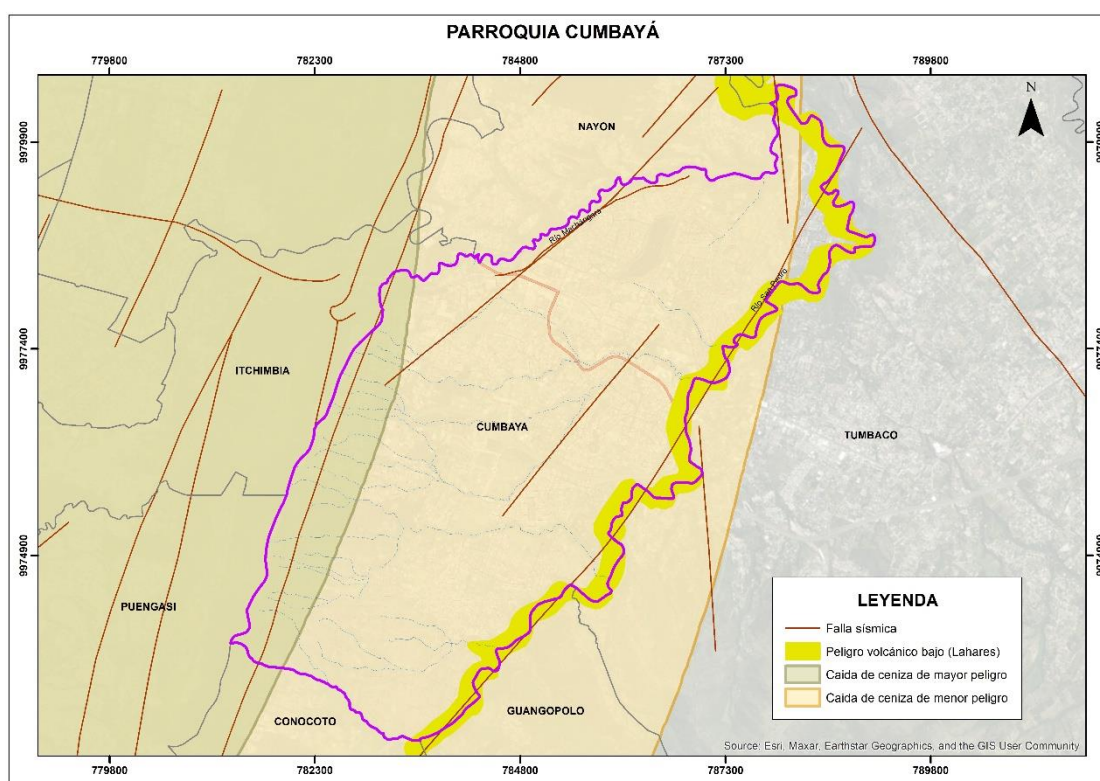
Mapa 6. Amenazas volcánicas y sísmicas
