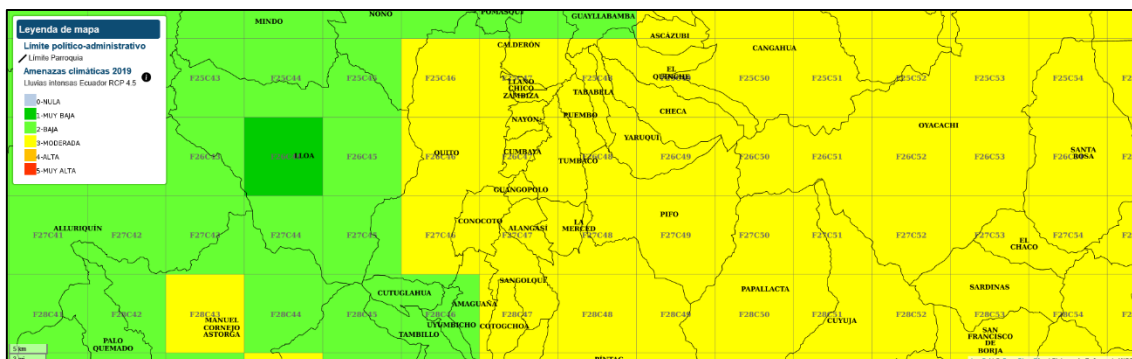
Ilustración 4. Amenaza para lluvias intensas. Escenarios RCP 8.5 2016 – 2040
